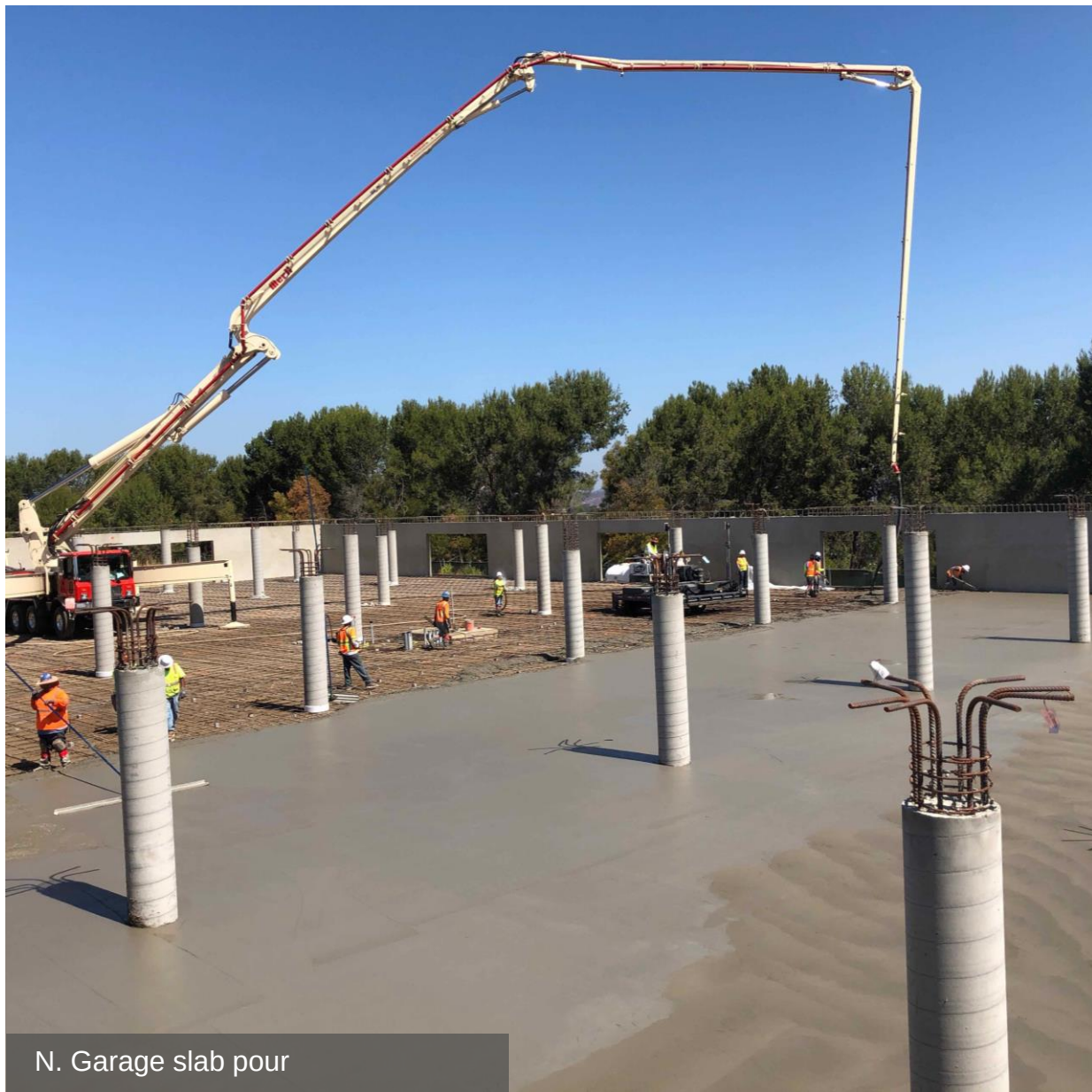
N. Garage slab pour
